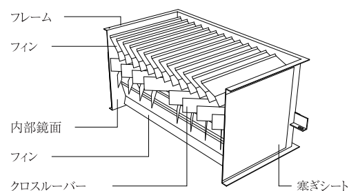
採光の仕組み（断面イメージ）
